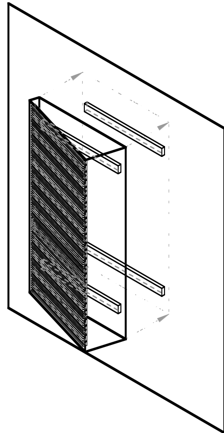
4 ISOMETRIC VIEW 05.00 Scale: 1:20
