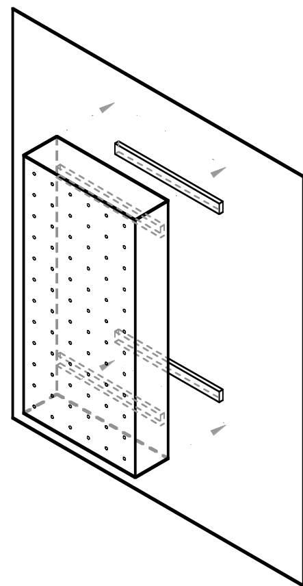
4 ISOMETRIC VIEW 03.00 Scale: 1:20
